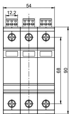
Габаритные размеры
